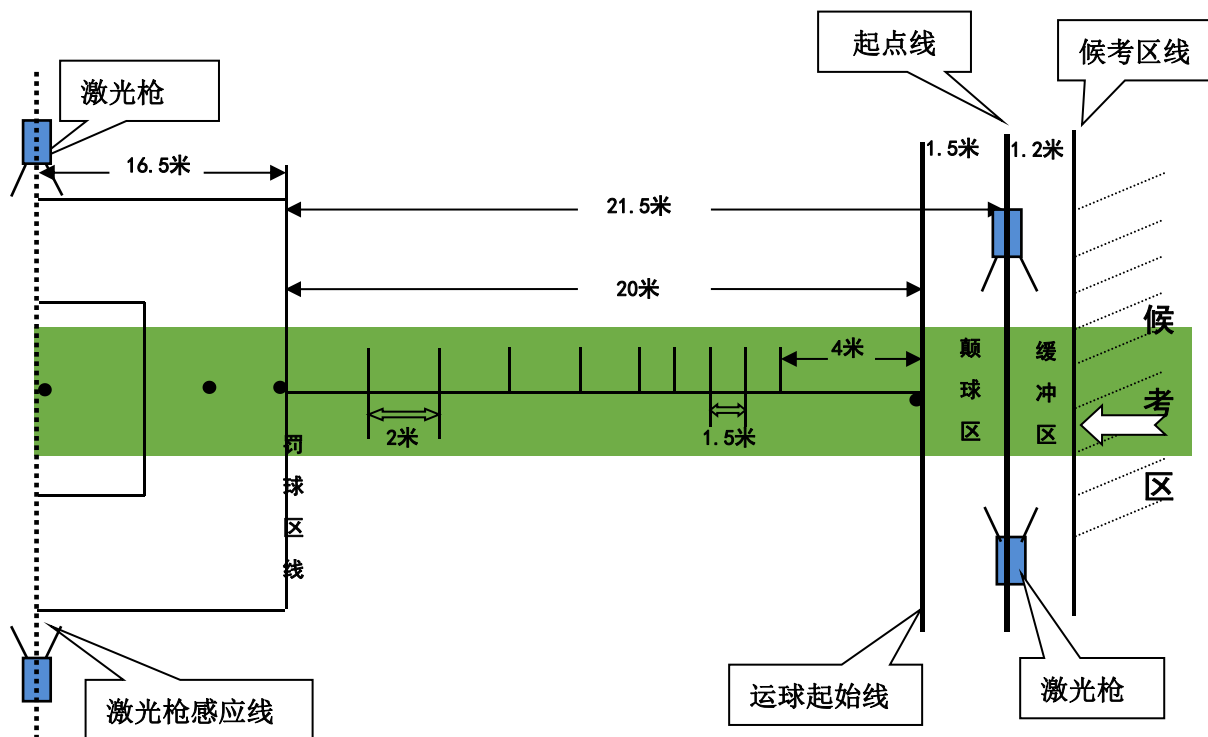
图7 足球运球绕杆射门场地图
